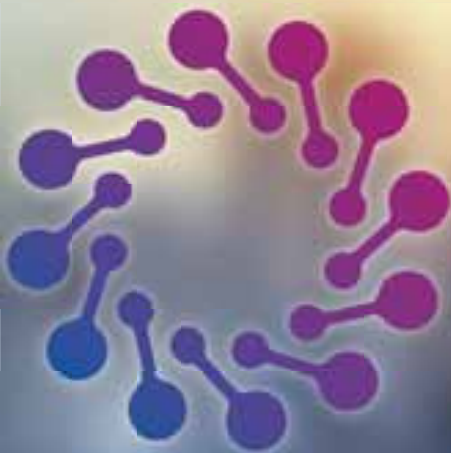
inteligentna fabryka
