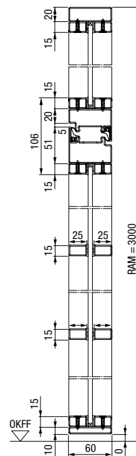
1-skrzydłowe stalowe drzwi loftowe z naświetlem górnym, przekrój pionowy
