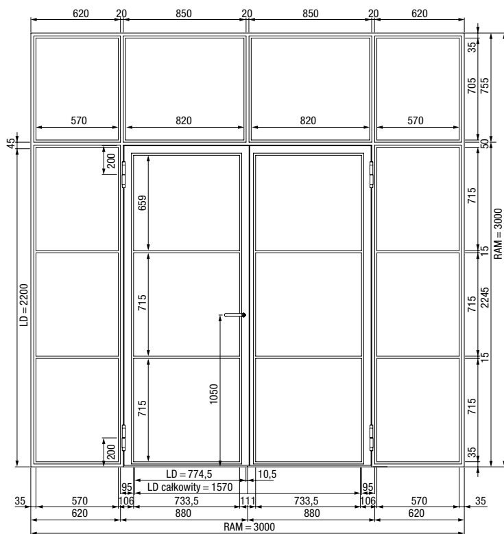
2-skrzydłowe stalowe drzwi loftowe z naświetlami bocznymi i naświetlem górnym
