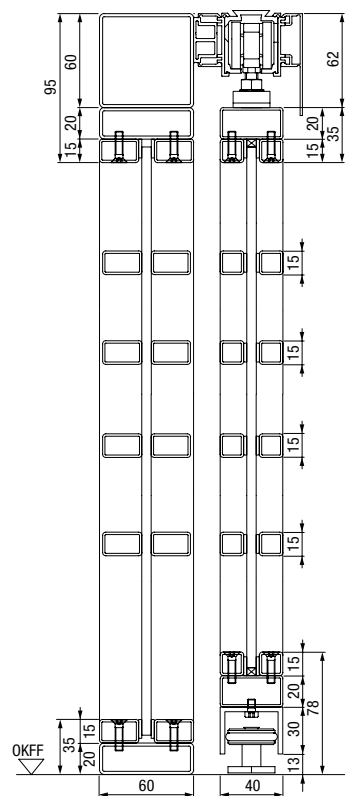
2-skrzydłowe stalowe drzwi loftowe z naświetlem bocznym, przekrój pionowy
