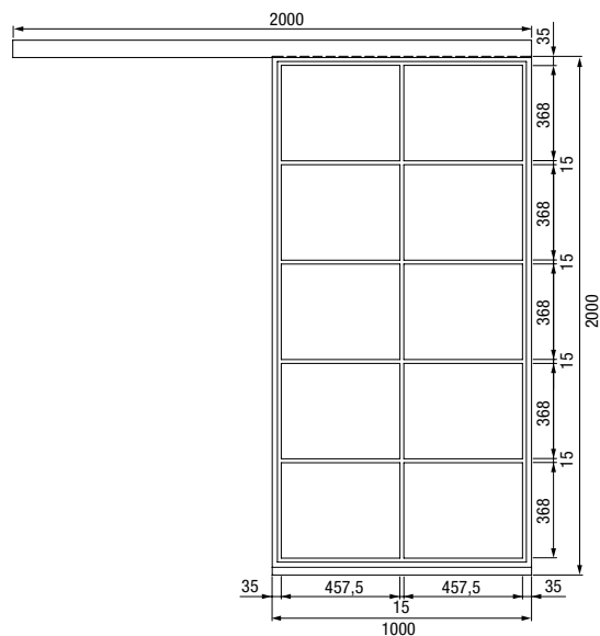
1-skrzydłowe stalowe drzwi loftowe
