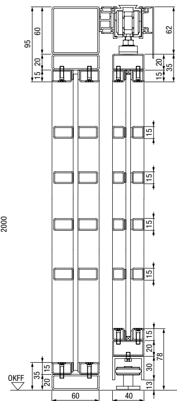
2-skrzydłowe stalowe drzwi loftowe z naświetlami bocznymi, przekrój pionowy
