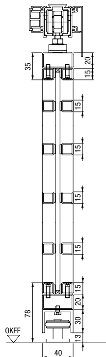
1-skrzydłowe stalowe drzwi loftowe, przekrój pionowy
