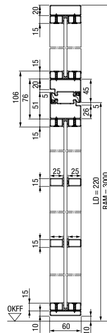
2-skrzydłowe stalowe drzwi loftowe z naświetlem górnym, przekrój pionowy
