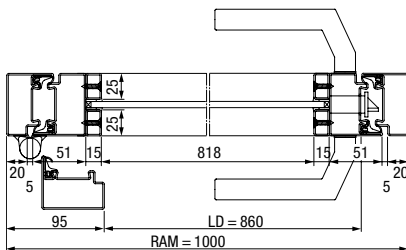
1-skrzydłowe stalowe drzwi loftowe, przekrój poziomy
