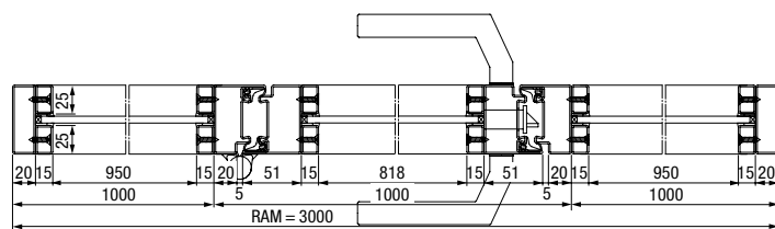
1-skrzydłowe stalowe drzwi loftowe z naświetlami bocznymi, przekrój poziomy
