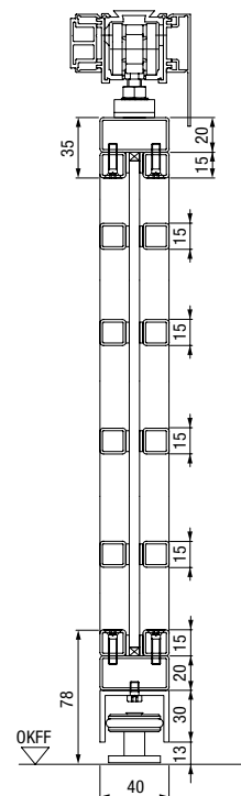
2-skrzydłowe stalowe drzwi loftowe, przekrój pionowy
