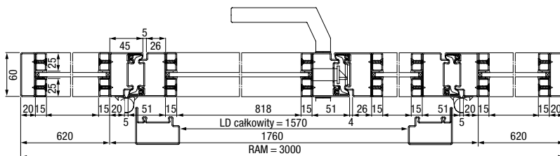
2-skrzydłowe stalowe drzwi loftowe z naświetlami bocznymi, przekrój poziomy
