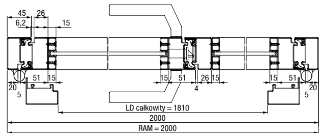
2-skrzydłowe stalowe drzwi loftowe, przekrój poziomy
