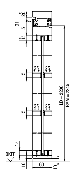
1-skrzydłowe stalowe drzwi loftowe, przekrój pionowy
