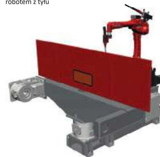
FRAME-IT+H ze stołem obrotowym i robotem z tyłu
