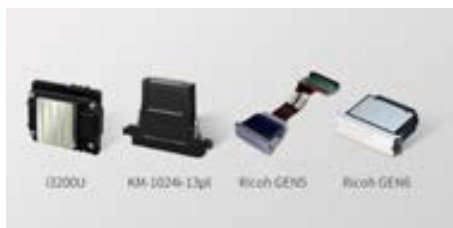
różne warianty głowic drukujących
